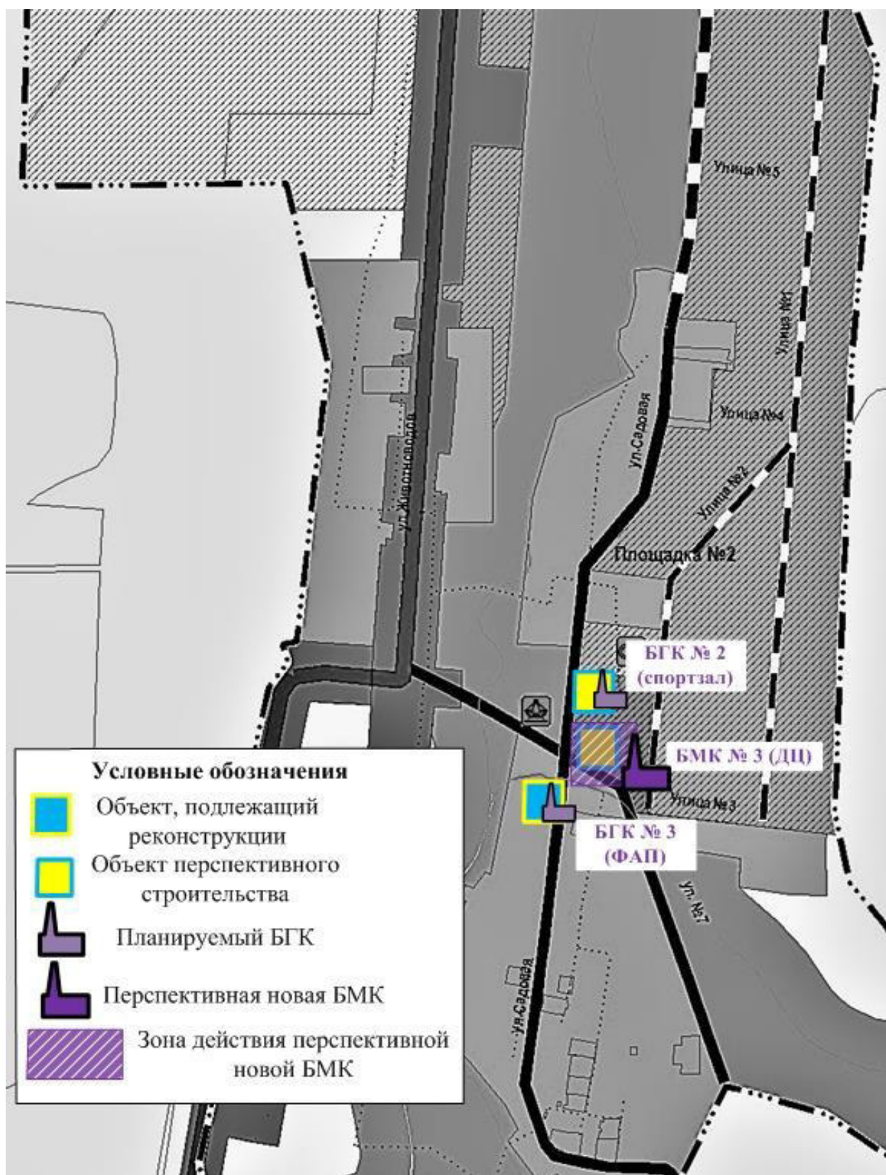
Рис. № 19 – Перспективные зоны теплоснабжения планируемых источников т. э. на территории поселка Малые Ключи
